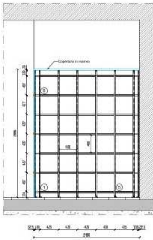
PROSPETTO FRONTALE STRUTTURA
